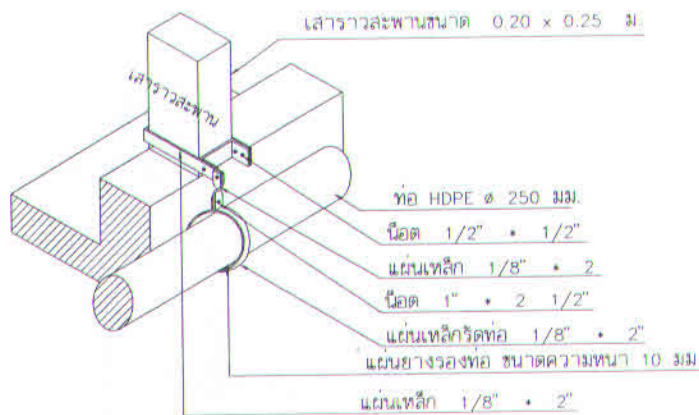
จุดยึดท่อกับสะพาน
